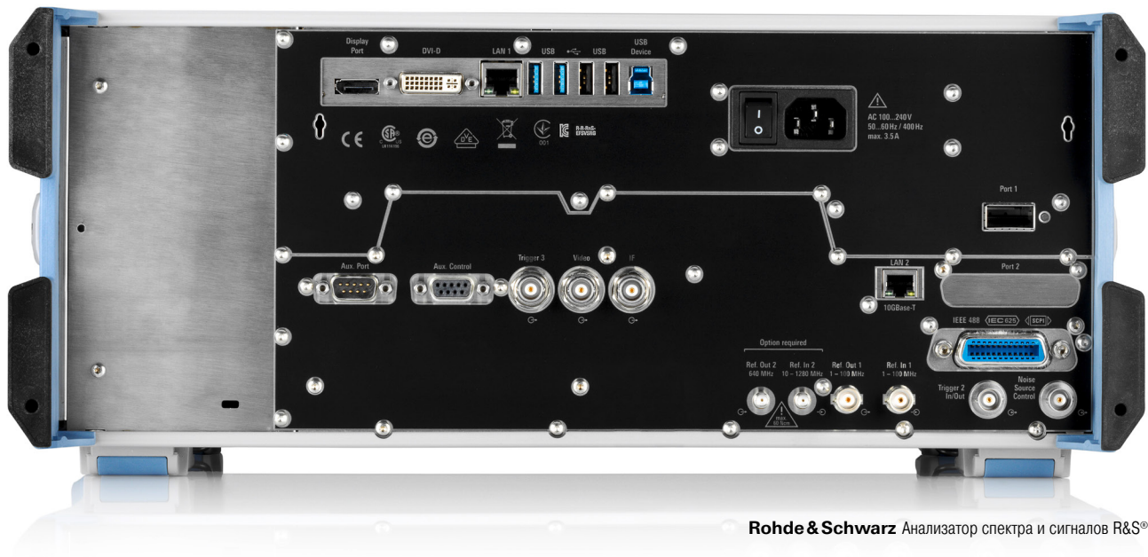
R&S®FSV3000: вид сзади
